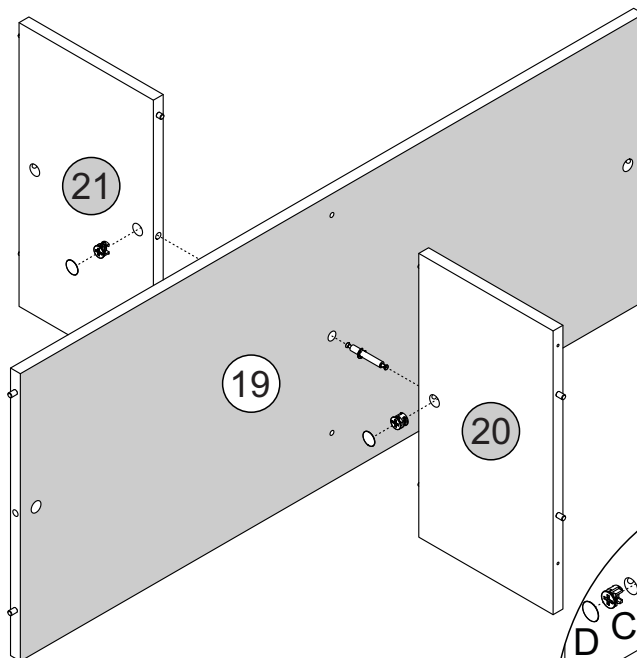
Detalhe 1 Detail/Detalle
