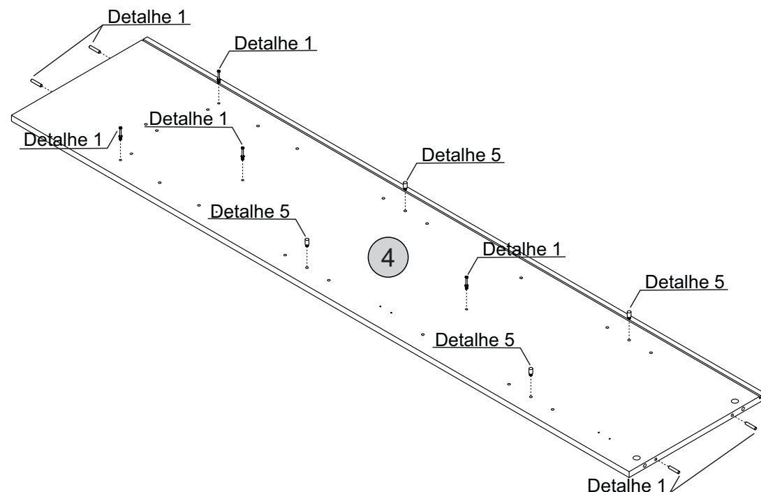
Detalhe 1 Detail/Detalle
