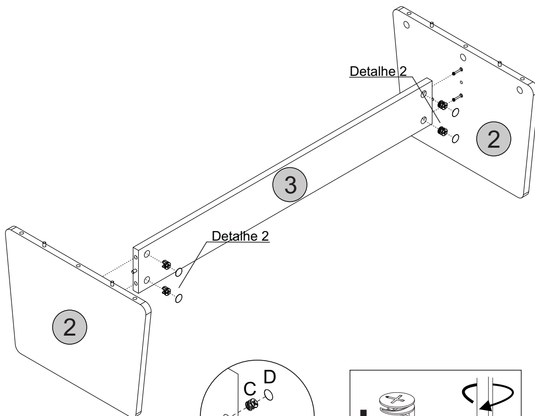
Detalhe 2 Detail/Detalle
