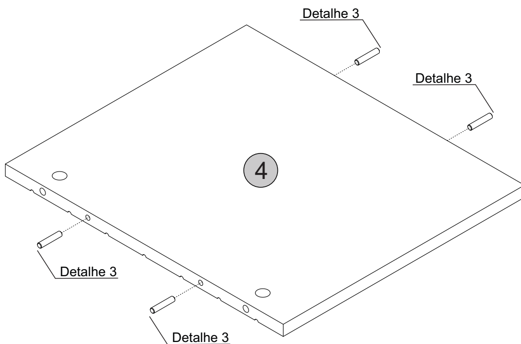
Detalhe 3 Detail/Détalle
