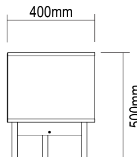
lateral/lado/side
