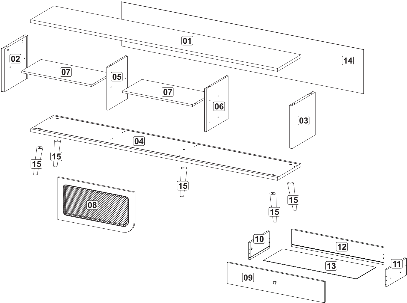
Vista de peças / Parts view / Vista de piezas
