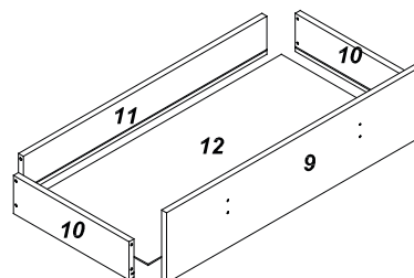
Móvel explodido
