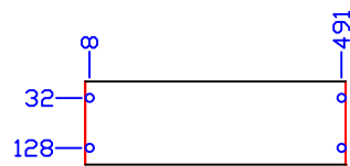
RODAPÉS FRONTAL E TRASEIRO 499x160
