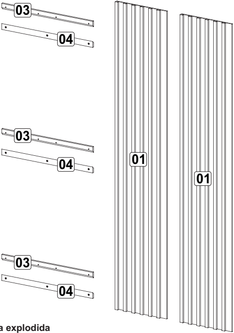
*Vista explodida
