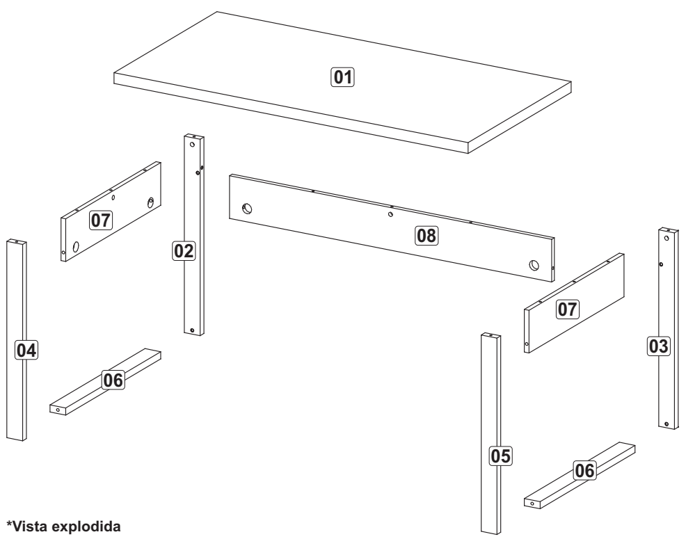
*Vista explodida
