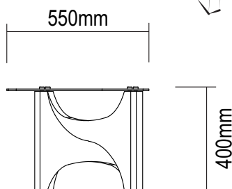
lateral/lado/side
