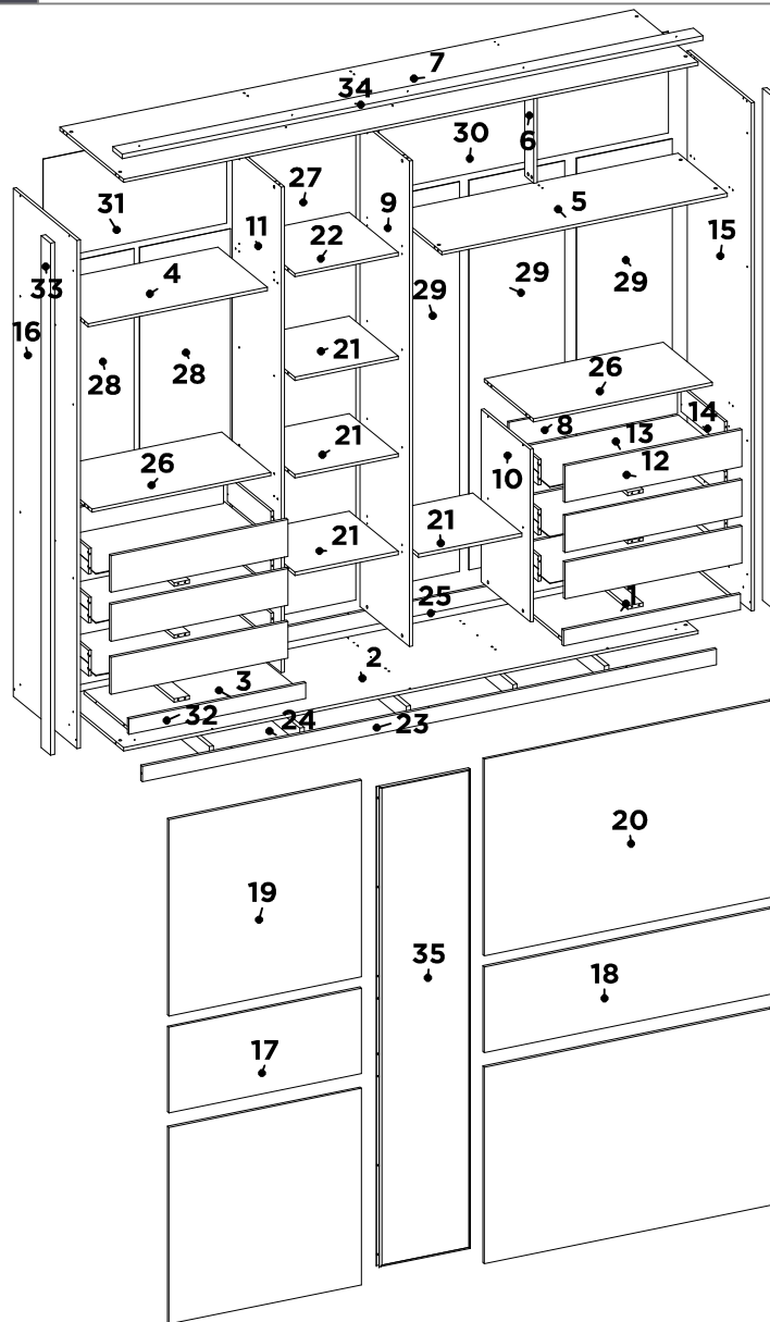
VISTA EXPLODIDA DO PRODUTO EXPLODED VIEW OF THE PRODUCT VISTA DESPIECE DEL PRODUCTO
