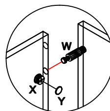
DETALHE MINIFIX
