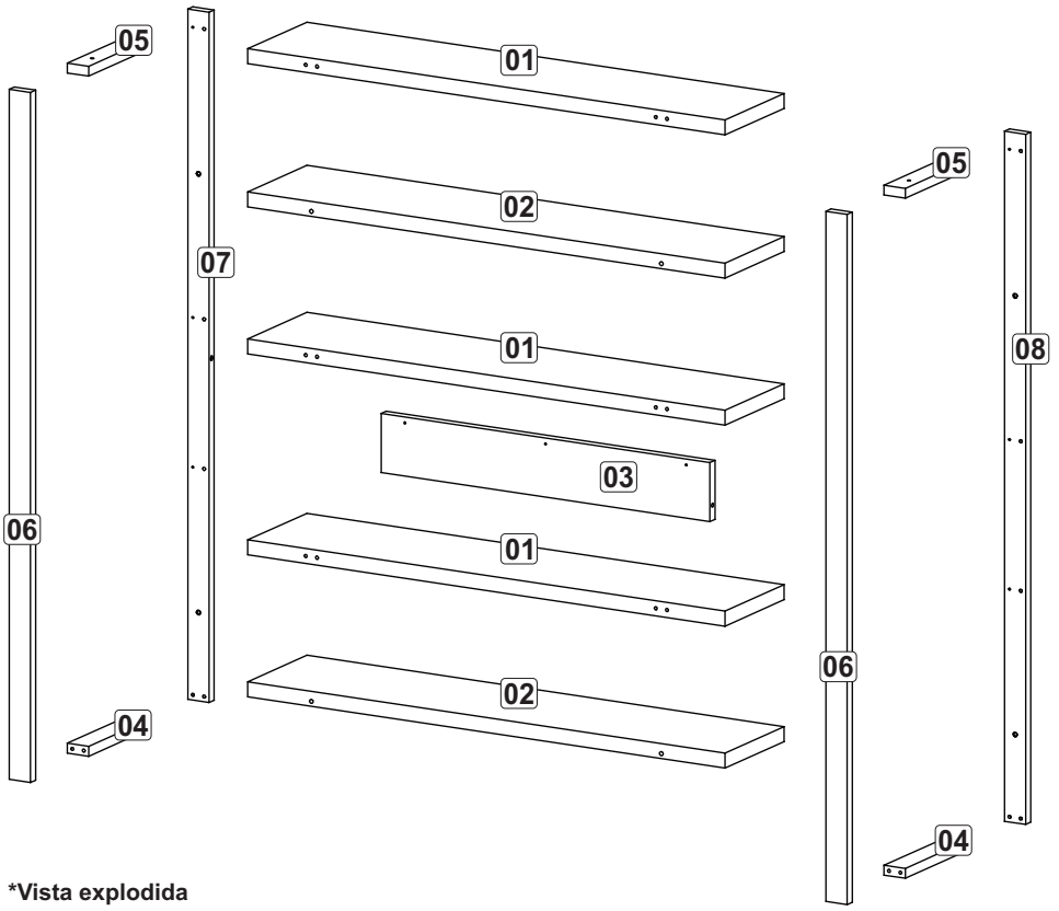
*Vista explodida
