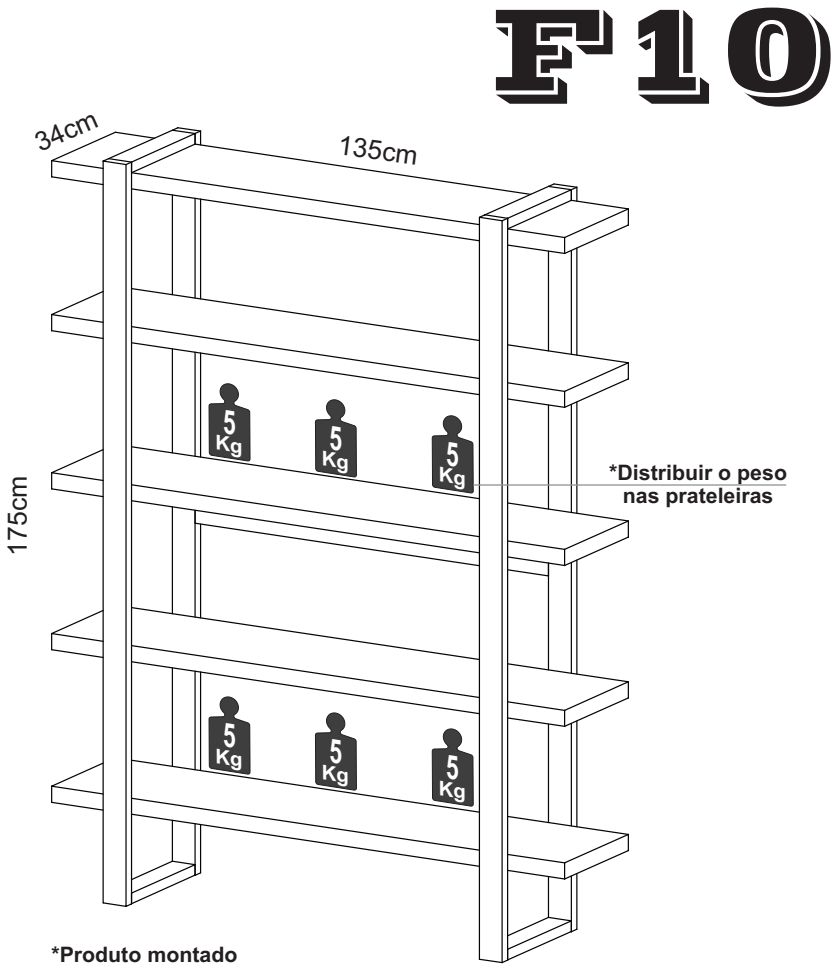
*Produto montado
