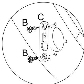
Detalhe 1 Detail/Detalle
