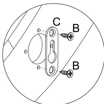
Detalhe 1 Detail/Detalle
