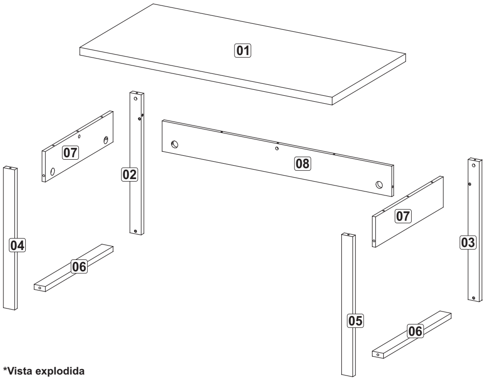
*Vista explodida
