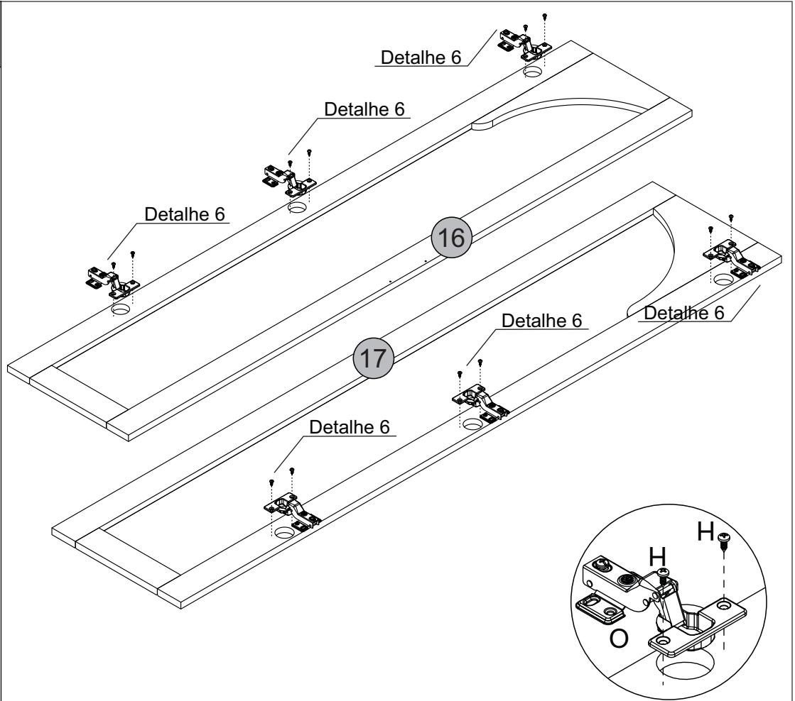
Detalhe 6 Detail/Detalle
