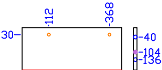
LATERAL DIREITA DO GAVETÃO 420x180 FURAR DE CIMA P/ BAIXO
