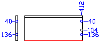
LATERAL ESQUERDA DO GAVETÃO 420x180 FURAR DE BAIXO P/ CIMA
