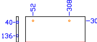
LATERAL ESQUERDA DO GAVETÃO 420x180 FURAR DE CIMA P/ BAIXO
