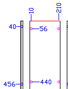
BASE 220x496 FURAR DE CIMA P/BAIXO
