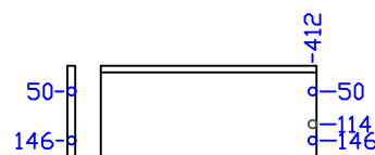
LATERAL ESQUERDA DO GAVETÃO 420x180
