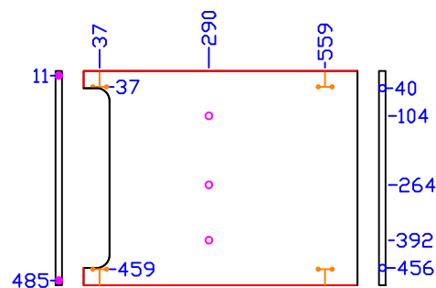
DIVISÓRIA 634x496 FURAR DE CIMA P / BAIXO
