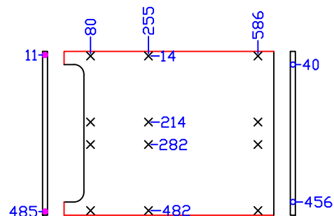
DIVISÓRIA 634x496 FURAR DE BAIXO P / CIMA
