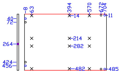
LATERAL DIREITA 720x496
