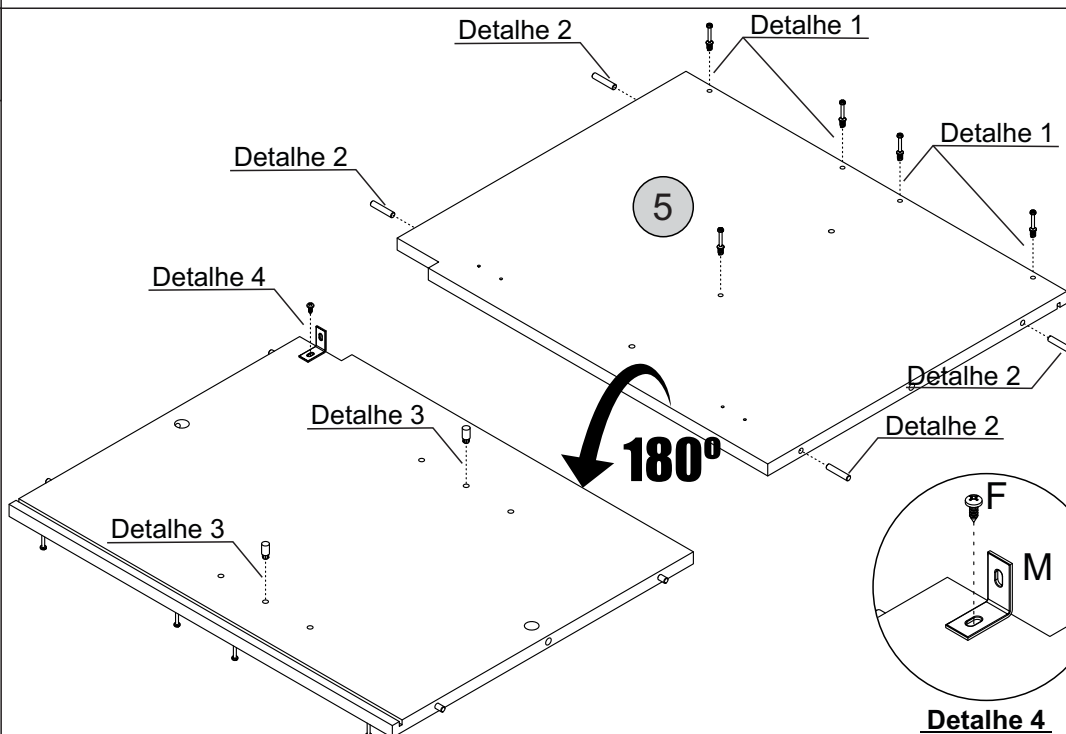
Detalhe 2 Detail/Detalle
