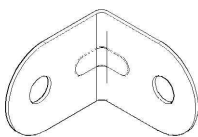
CANTONEIRA 18X18X14 (06)
