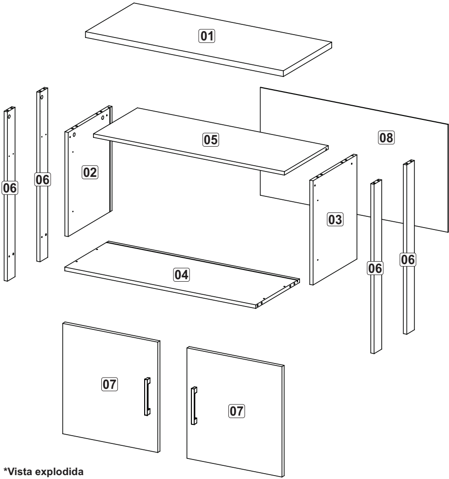
*Vista explodida
