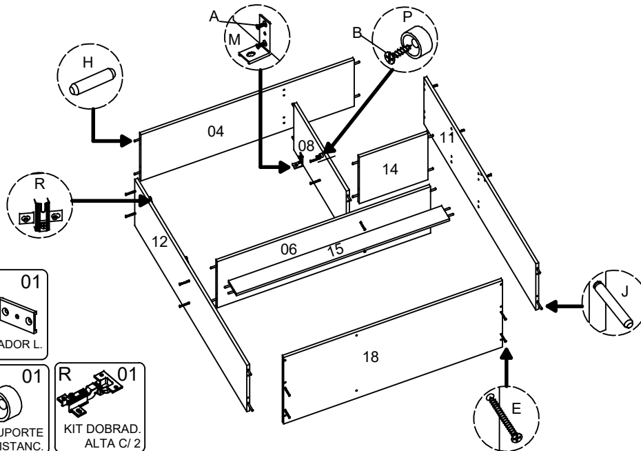
② MONTAGEM DA ESTRUTURA SUPERIOR. UPPER STRUCTURE ASSEMBLY. MONTAJE DE LA ESTRUCTURA SUPERIOR.
