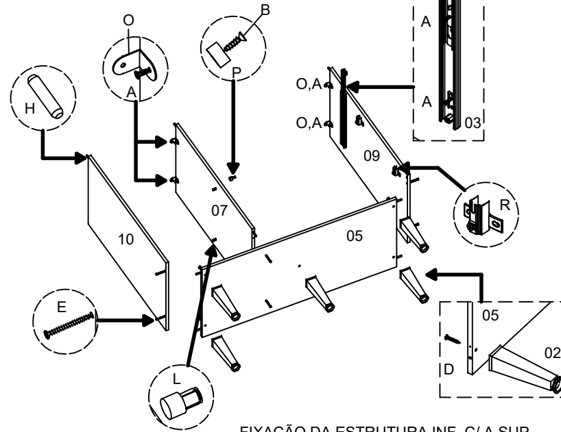
③ FIXAÇÃO DA ESTRUTURA INF. C/ A SUP. UPPER STRUCTURE ATTACHMENT INTO LOWER. FIJACIÓN DE LA ESTRUCTURA INF. CON LA SUP.
