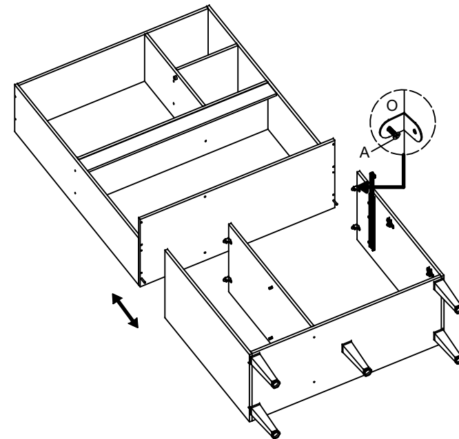
③ FIXAÇÃO DA ESTRUTURA INF. C/ A SUP. UPPER STRUCTURE ATTACHMENT INTO LOWER. FIJACIÓN DE LA ESTRUCTURA INF. CON LA SUP.
