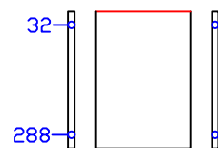
PRATELEIRAS 220x320 2 PEÇAS
