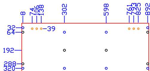
LATERAIS 900x352 2 PEÇAS
